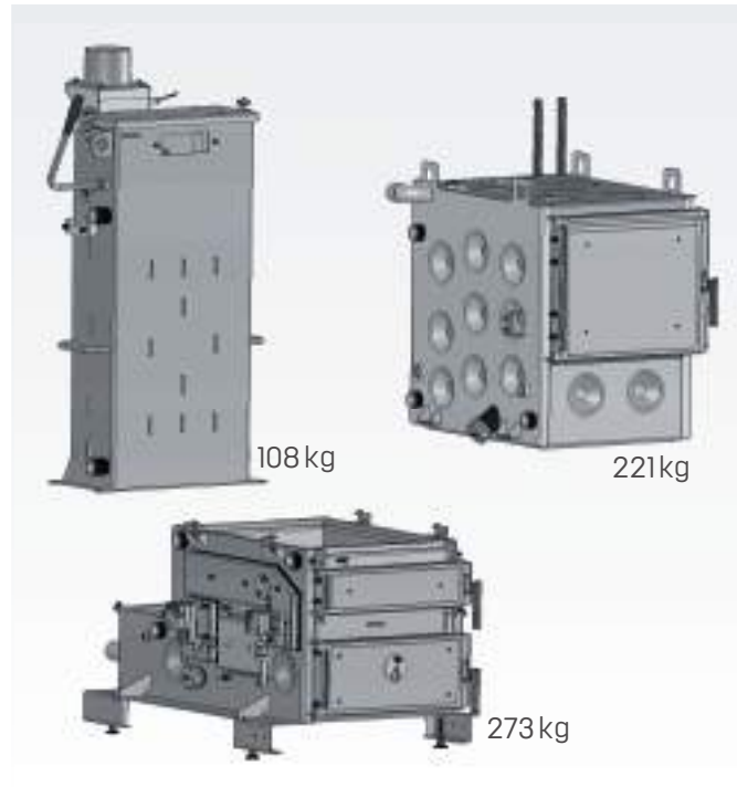
KWB Classicfire – pannan kan demonteras i tre delar.
